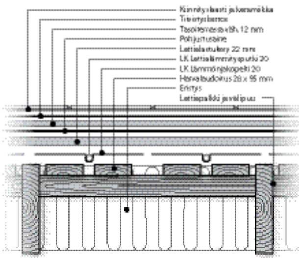
LK Lämmönjakopelti 20 asennettuna harvalaudoitukseen lattiapalkkien väliin. Keraamiset laatat märkätiloissa.
