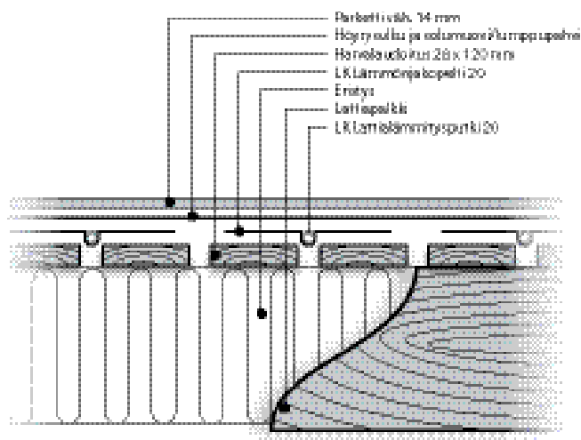
Lämmönjakopelti 20 asennettuna harvalaudoitukseen lattiapalkkien päälle. Lattiamateriaali parkettia.
