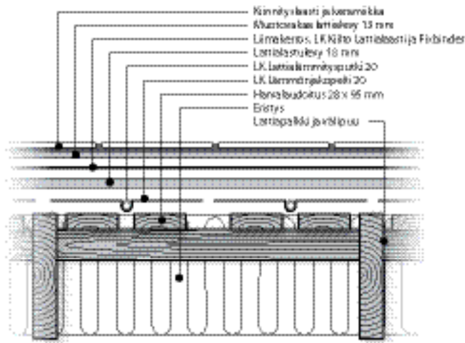
LK Lämmönjakopelti 20 asennettuna harvalaudoitukseen lattiapalkkien väliin. Keraamiset laatat kuivatiloissa.
